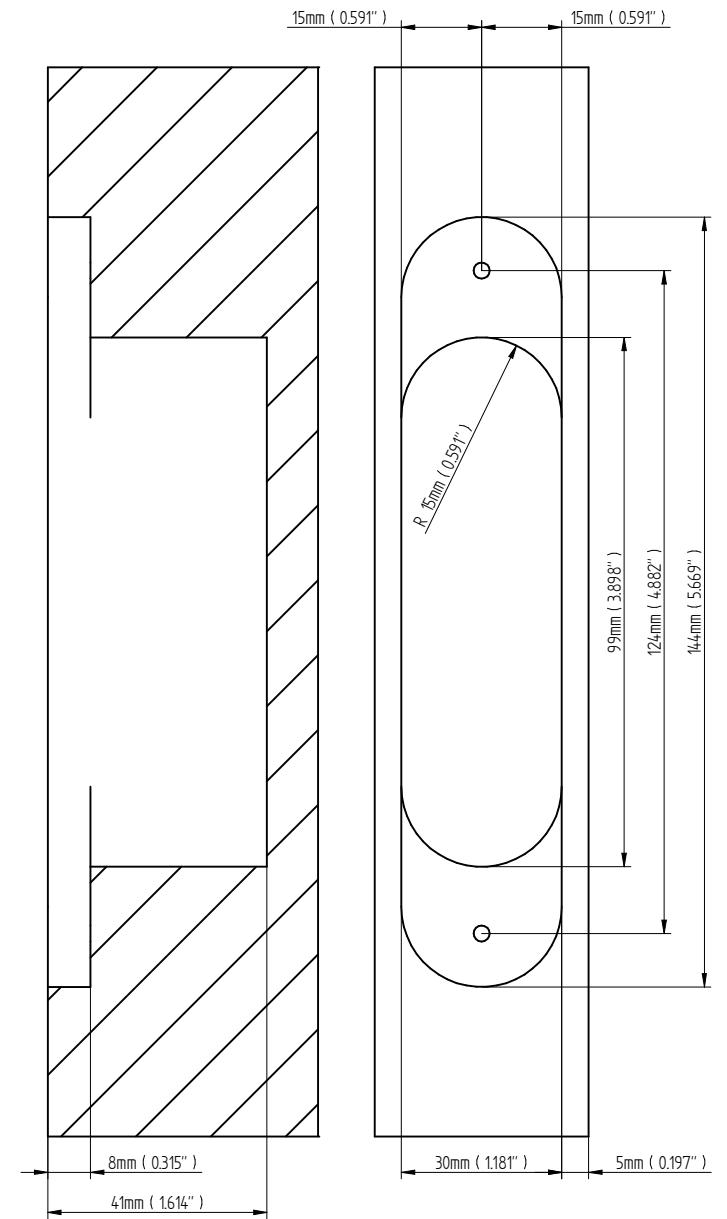
Template door panel
